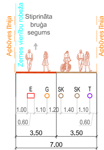
Šķēršprofils 3-3
