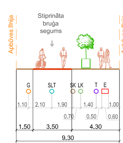
Šķēršprofils 4-4
