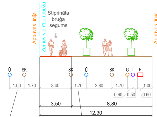
Šķēršprofils 1-1
