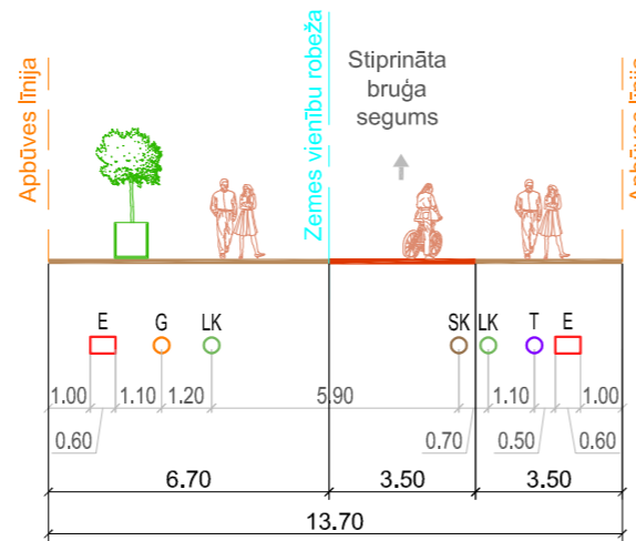
Šķēršprofils 2-2
